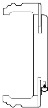
Futterbrett mit Rundkante
